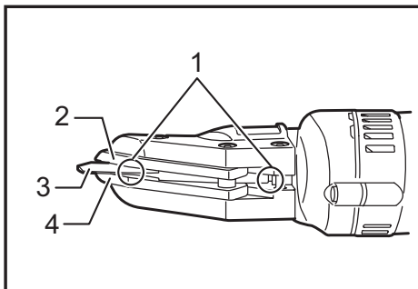
► 1. Lubrifier 2. Lame latérale G 3. Lame centrale 4. Lame latérale D
