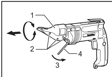
► 1. Tête de coupe 2. Vis 3. Desserrer 4. Clé hexagonale
