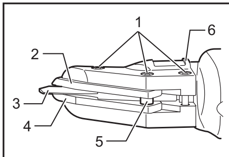
► 1. Vis 2. Lame latérale G 3. Lame centrale 4. Lame latérale D 5. Manchon 6. Tête de coupe
