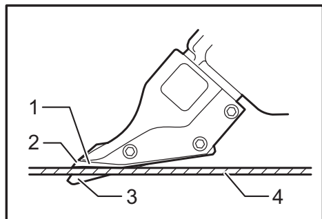
► 1. Surface de la lame latérale 2. Lames latérales 3. Lame centrale 4. Pièce
