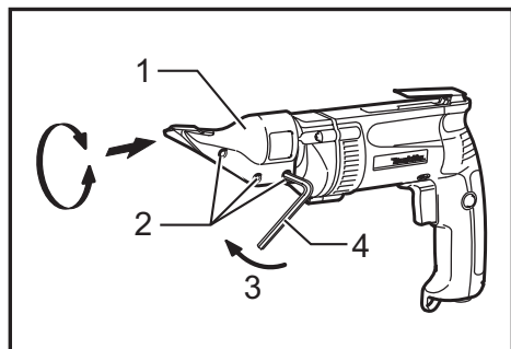
► 1. Tête de coupe 2. Vis 3. Serrer 4. Clé hexagonale
