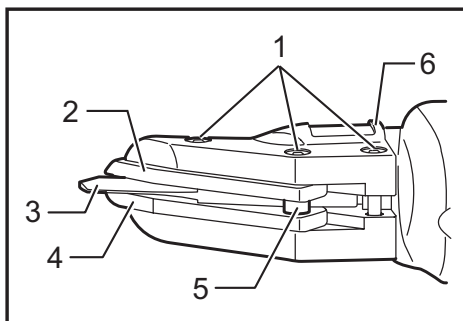
► 1. Tornillos 2. Cuchilla lateral izquierda (L) 3. Superficie de cuchilla central 4. Cuchilla lateral derecha (R) 5. Base de mandril 6. Cabeza cortadora
