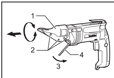
► 1. Cabeza cortadora 2. Tornillos 3. Aflojar 4. Llave hexagonal
