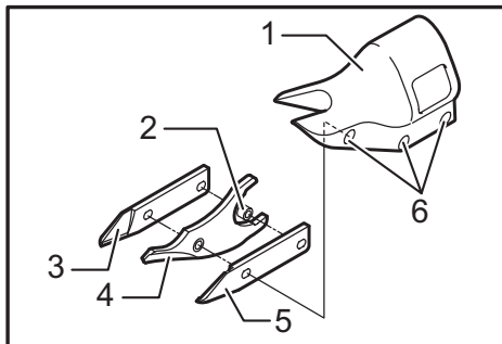
► 1. Tête de coupe 2. Manchon 3. Lame latérale D 4. Lame centrale 5. Lame latérale G 6. Vis
